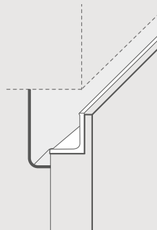
Gola "Elle" Profilo art. 485
